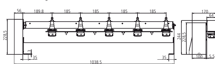
SK 30 tool changer
