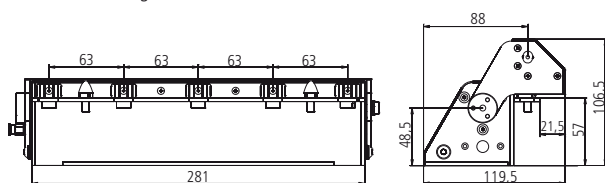
SK 11 tool changer
